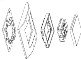
Zentralplatte, Designrahmen (nicht im Lieferumfang enthalten), Zwischenrahmen, Wandsender, Betätigungswippe(n)
